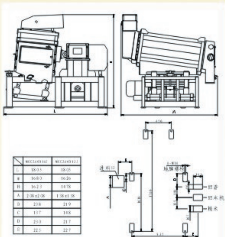
(外形尺寸与地脚安装图)
